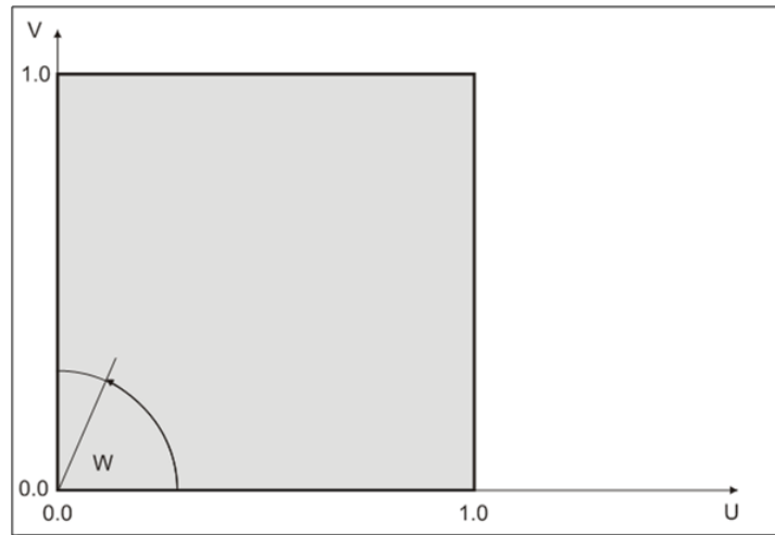
Abbildung 1: U-V-Koordinatenraum
