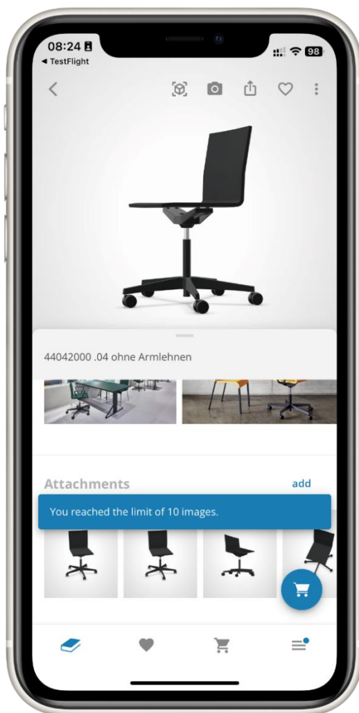
Figure 2 - Hinweismeldung
